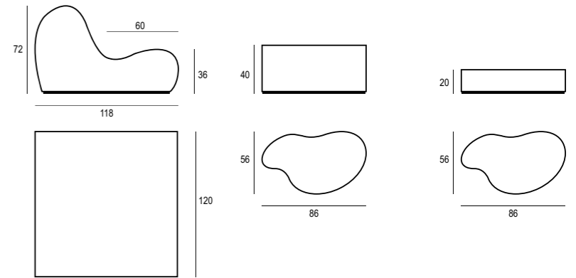
LAND.6 divano due posti 2 seater sofa peso indicativo 65 kg
