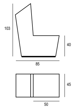
CUT.2 seduta seat peso indicativo 28 kg
