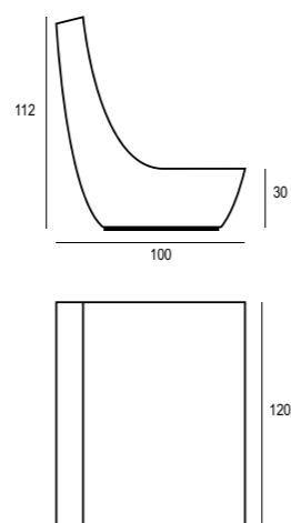
COMMA.2 divano 2 posti 2 seater sofa peso indicativo 62 kg
