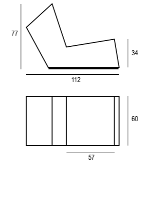
CUT.3.60 poltrona arm chair peso indicativo 38 kg
