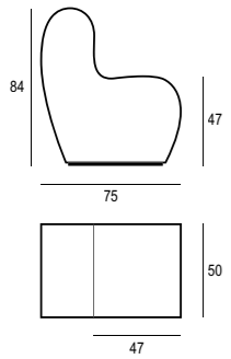
LAND.1 seduta seat peso indicativo 25 kg
