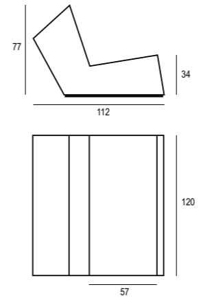
CUT.3.120 divano due posti 2 seater sofa peso indicativo 58 kg
