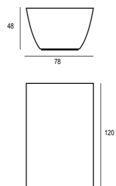
COMMA.5 tavolino table peso indicativo 36 kg
