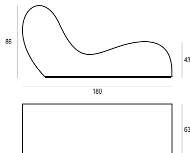
LAND.4 chaise longue peso indicativo 54 kg
