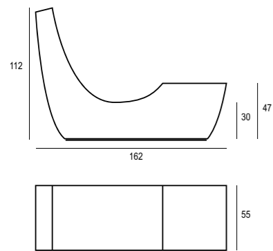
COMMA.1 chaise longue peso indicativo 50 kg
